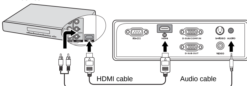
AV device
