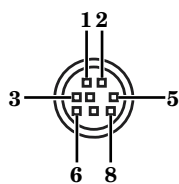
RS-232C (8P)
