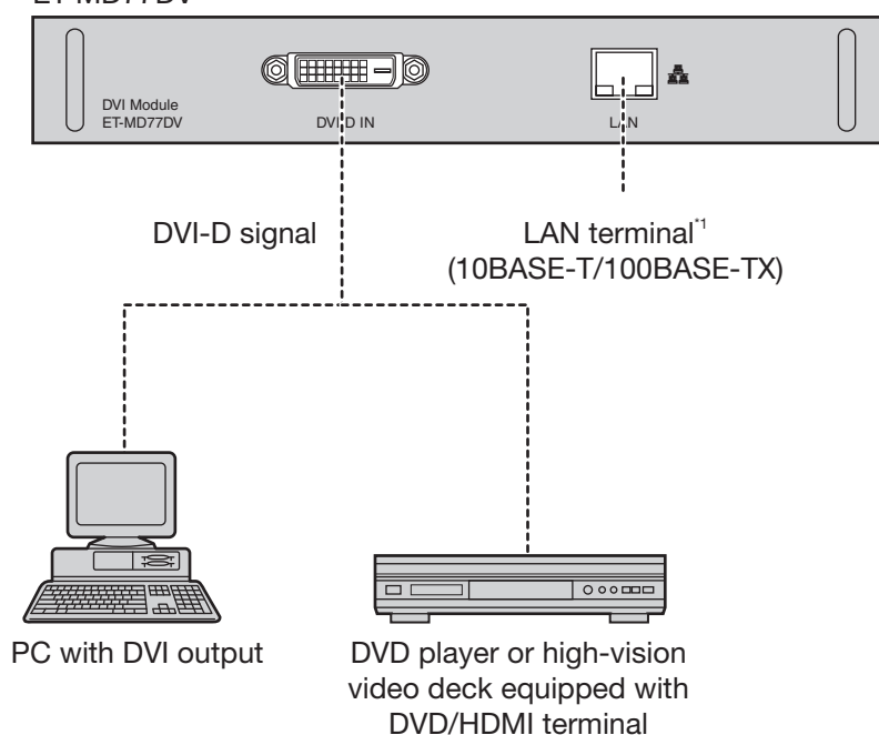
DVI-D input module (optional) ET-MD77DV
