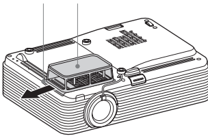
Luftfilterabdeckung Staubschutz
