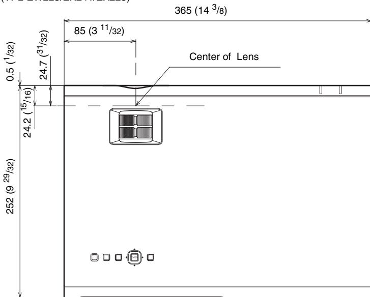
Top (VPL-EW225/EX241/EX225)
