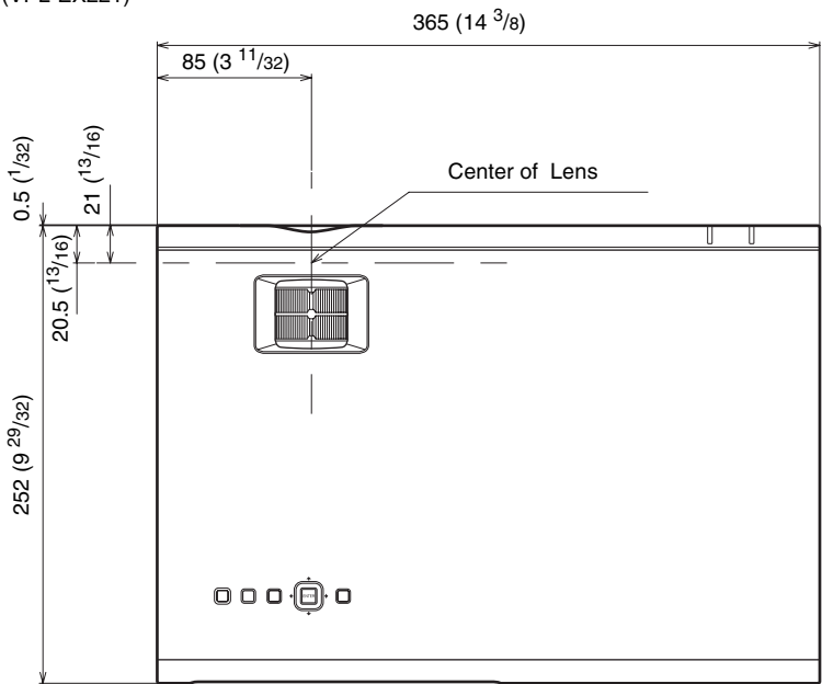
Top (VPL-EX221)
