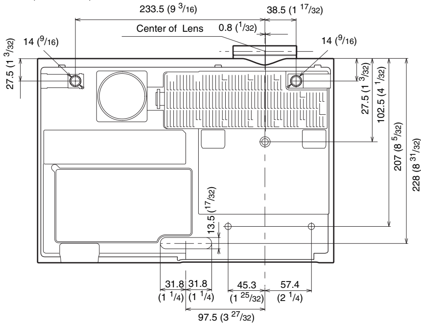
Bottom (VPL-EW275)
