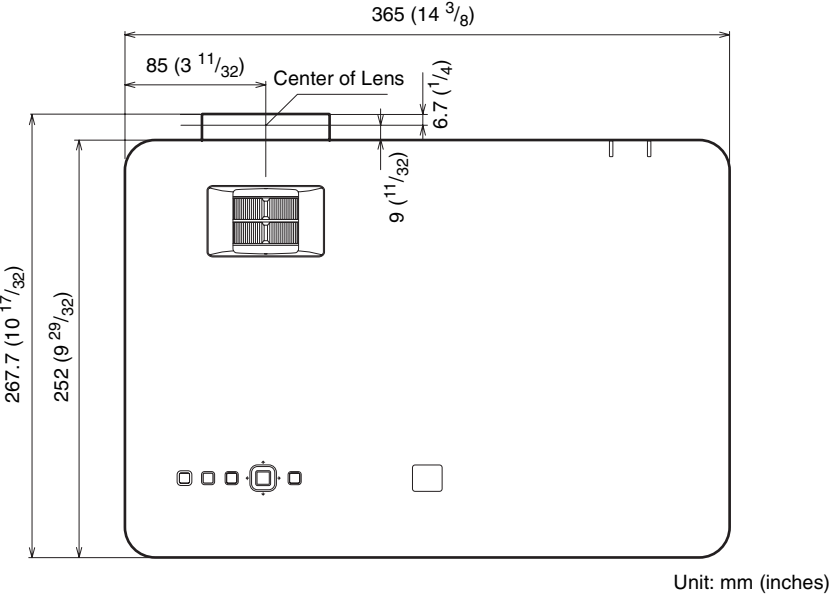
Top (VPL-EW348/EW345/EW315)
